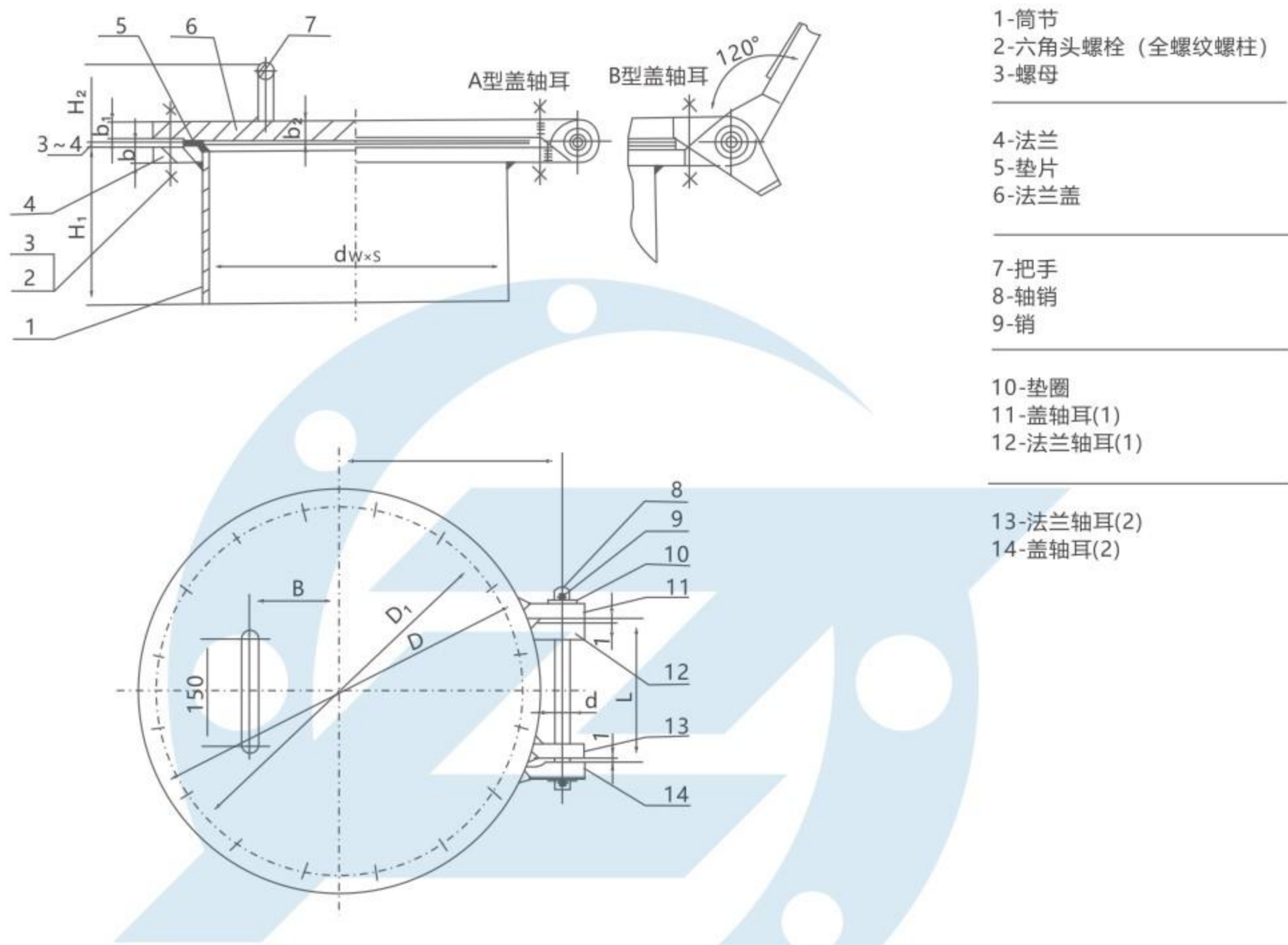
回旋盖板式平焊法兰人孔的型式尺寸
